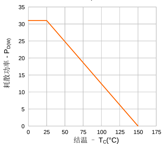
图13-2. 耗散功率vs.温度(SVS65R400FJH/FJDE3)
