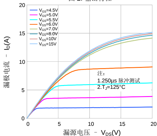
图 2. 输出特性
