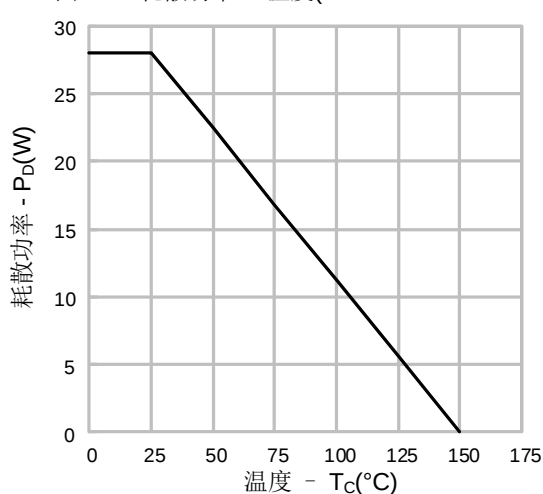
图14-1. 耗散功率vs.温度(SVSP65R180FJDD4)
