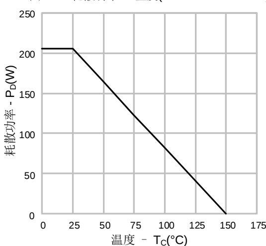
图14-2. 耗散功率vs.温度(SVSP65R180P7D4)
