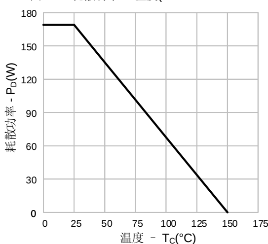
图14-3. 耗散功率vs.温度(SVSP65R180L8AD4)
