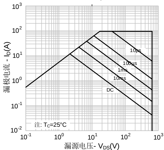
图 13-3. 最大安全工作区域(SVSP65R180L8AD4)
