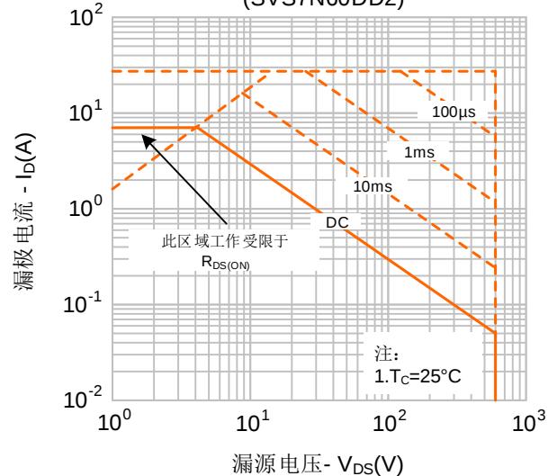
图 9-2 最大安全工作区域 (SVS7N60DD2)
