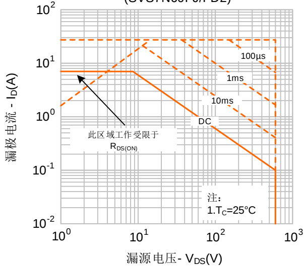
图 9-1.最大安全工作区域 (SVS7N60FJ/FD2)
