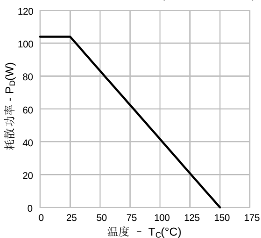
图14-2. 耗散功率vs.温度(SVS60R340DD4)
