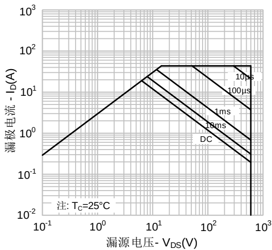
图 13-3. 最大安全工作区域(SVS60R340SD4)
