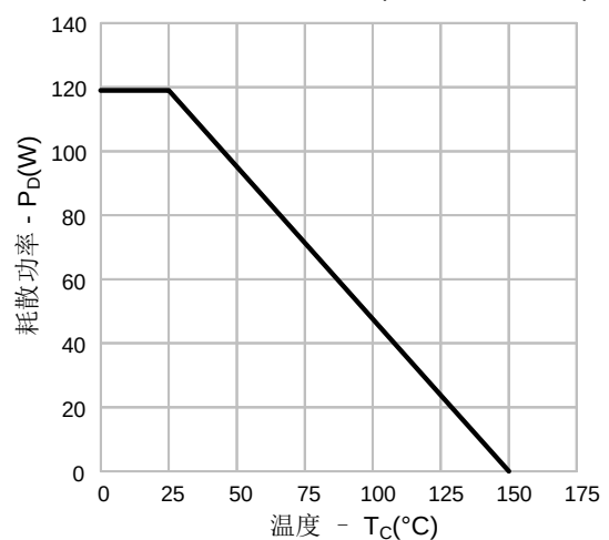
图14-3. 耗散功率vs.温度(SVS60R340SD4)
