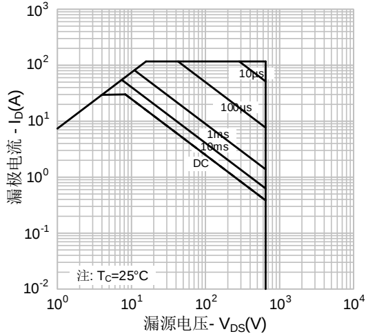
图 13-3. 最大安全工作区域(SVSP65R135L8AD4)
