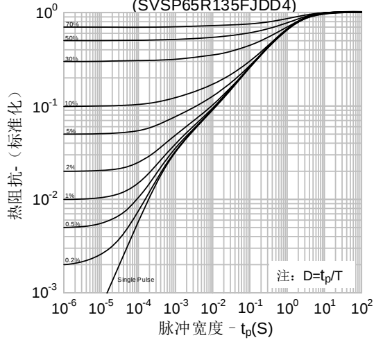
图16-2.瞬态热阻抗 vs. 脉冲宽度 (SVSP65R135FJDD4)
