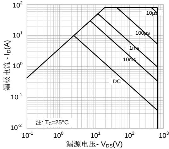
图 13-3. 最大安全工作区域(SVSP65R240L8AD4)
