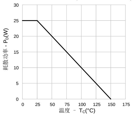
图14-3. 耗散功率vs.温度(SVSP65R240L8AD4)
