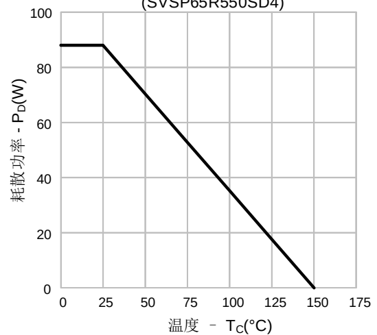
图14-3. 耗散功率vs.温度 (SVSP65R550SD4)
