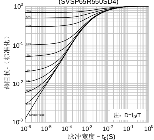
图16-3.瞬态热阻抗 vs. 脉冲宽度 (SVSP65R550SD4)
