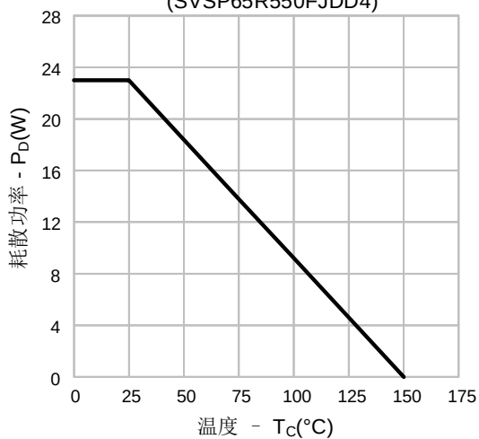
图14-2. 耗散功率vs.温度 (SVSP65R550FJDD4)
