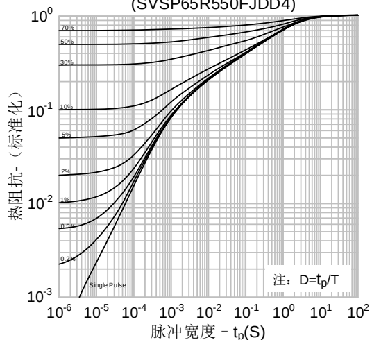
图16-2.瞬态热阻抗 vs. 脉冲宽度 (SVSP65R550FJDD4)
