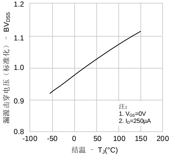
图7. 击穿电压vs.温度特性
